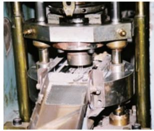
▲全自動粉末成形機は総数30台。精密な金型で金属の粉末がプレスされ、小さな部品が続々と成形されていく
